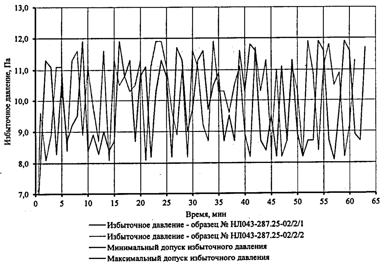
Рисунок 14. График избыточного давления в огневом пространстве печи при испытании
