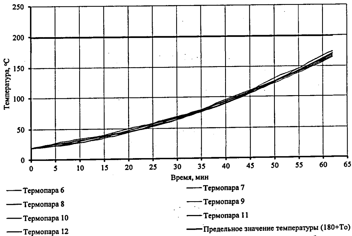
Рисунок 8. График изменения температуры на необогреваемой поверхности полотна образца № НЛ043-287.25-02/1/1
