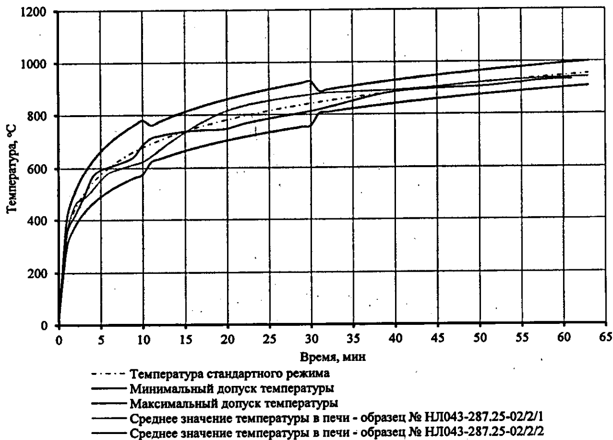
Рисунок 13. График изменения температуры во времени в огневой камере печи при испытании
