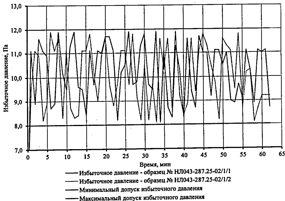
Рисунок 6. График избыточного давления в огневом пространстве печи при испытании
