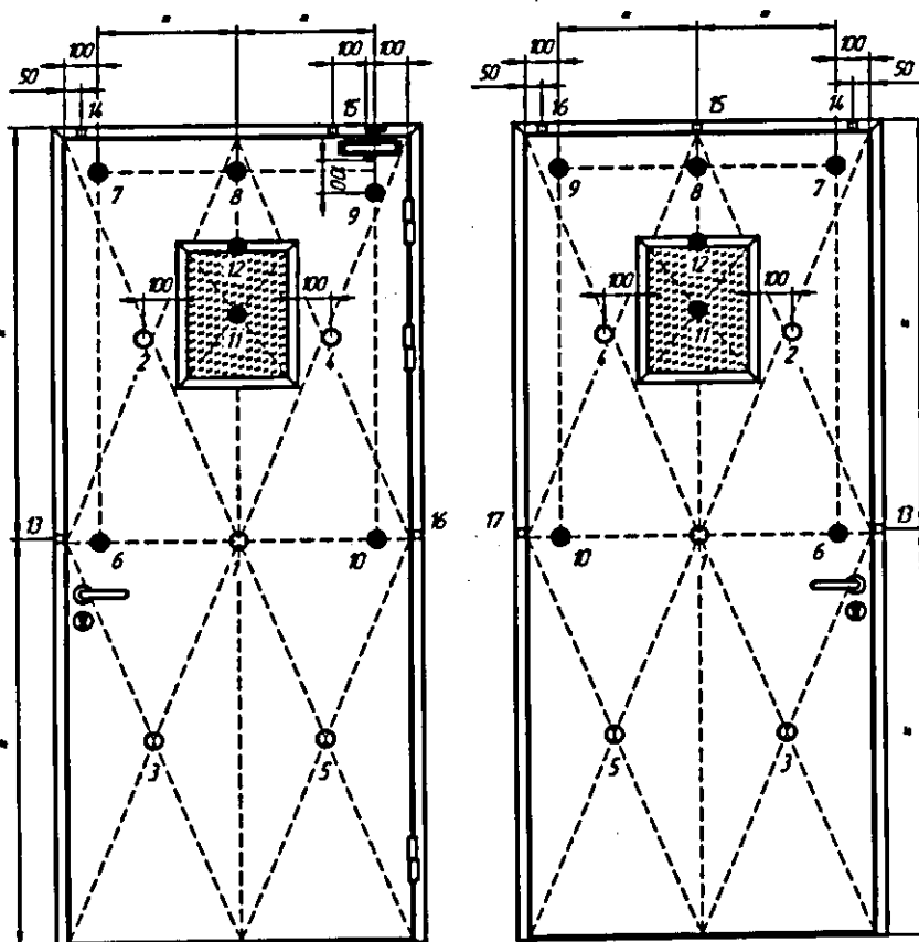
Рисунок 3. Схема установки термодпар на необогреваемой поверхности дверей деревянных противопожарных ДДПО-01-Е160 2550х1100
