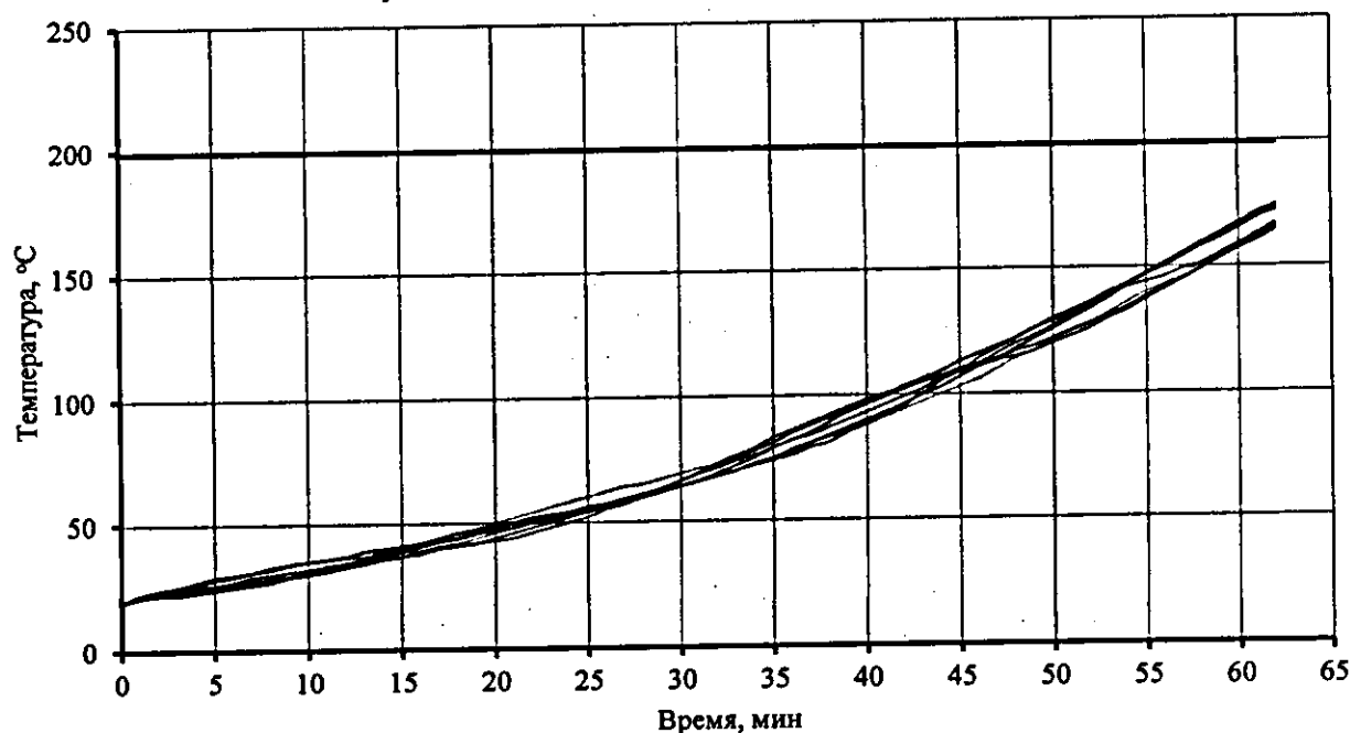
Рисунок 10. График изменения температуры и среднего значения температуры на необогреваемой поверхности полотна образца № НЛ043-287.25-02/1/2
