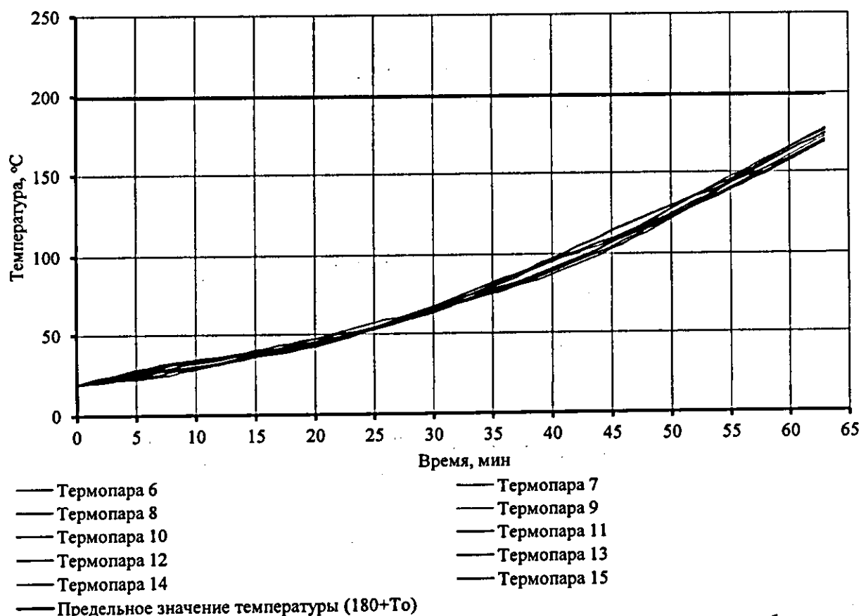
Рисунок 16. График изменения температуры на необогреваемой поверхности полотна образца № НЛ043-287.25-02/2/1
