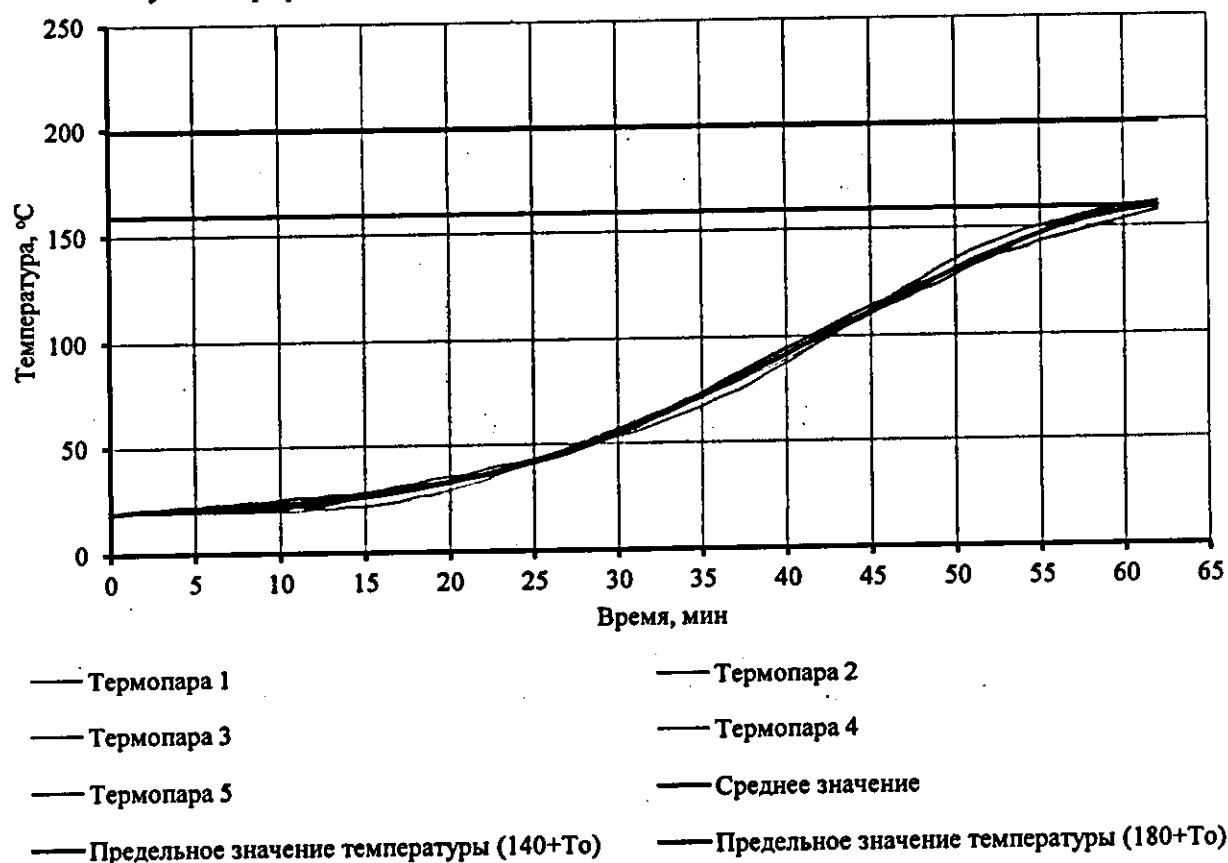
Рисунок 7. График изменения температуры и среднего значения температуры на необогреваемой поверхности полотна образца № НЛ043-287.25-02/1/1
