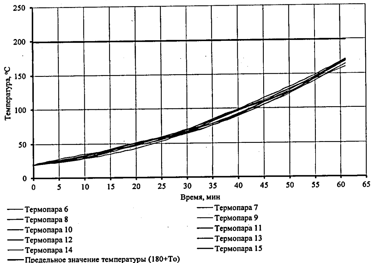
Рисунок 19. График изменения температуры на необогреваемой поверхности полотна образца № НЛ043-287.25-02/2/2
