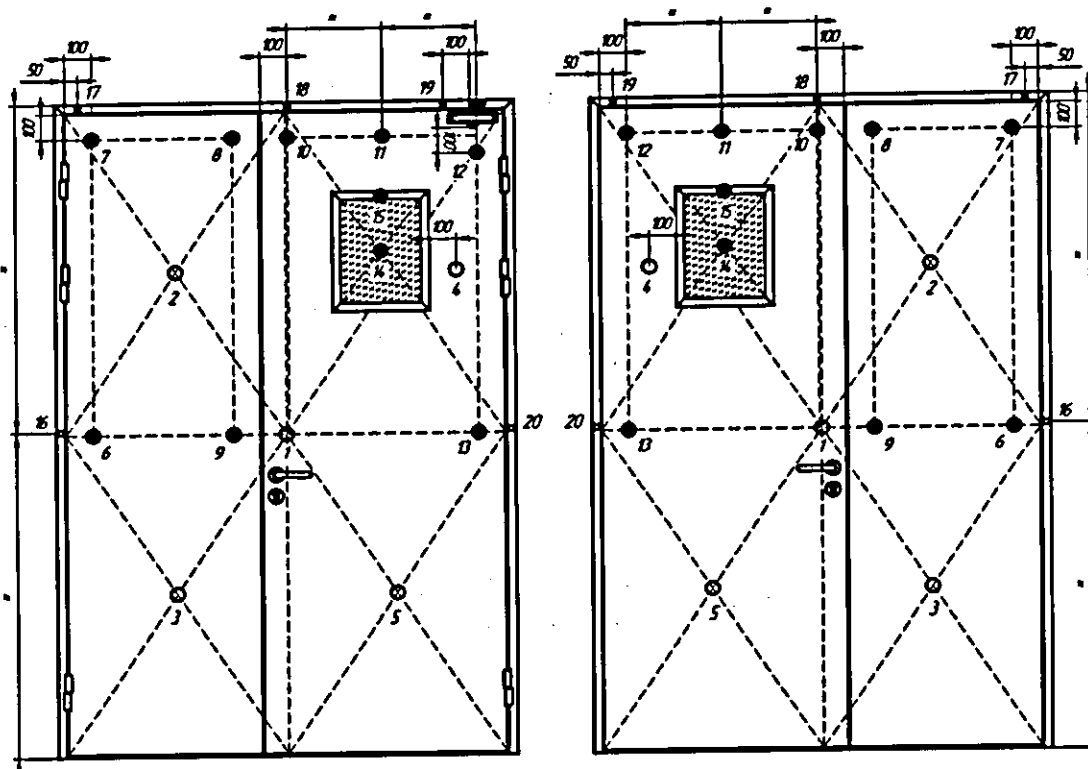
Рисунок 4. Схема установки термодпар на необогреваемой поверхности дверей деревянных противопожарных ДДПО-02-Е160 2550х1700
