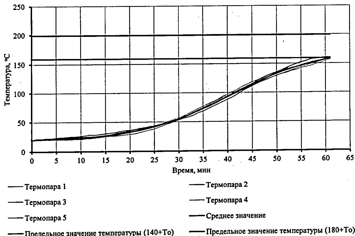
Рисунок 18. График изменения температуры и среднего значения температуры на необогреваемой поверхности полотна образца № НЛ043-287.25-02/2/2
