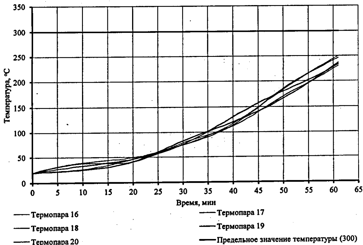
Рисунок 20. График изменения температуры на необогреваемой поверхности коробки образца № НЛ043-287.25-02/2/2
