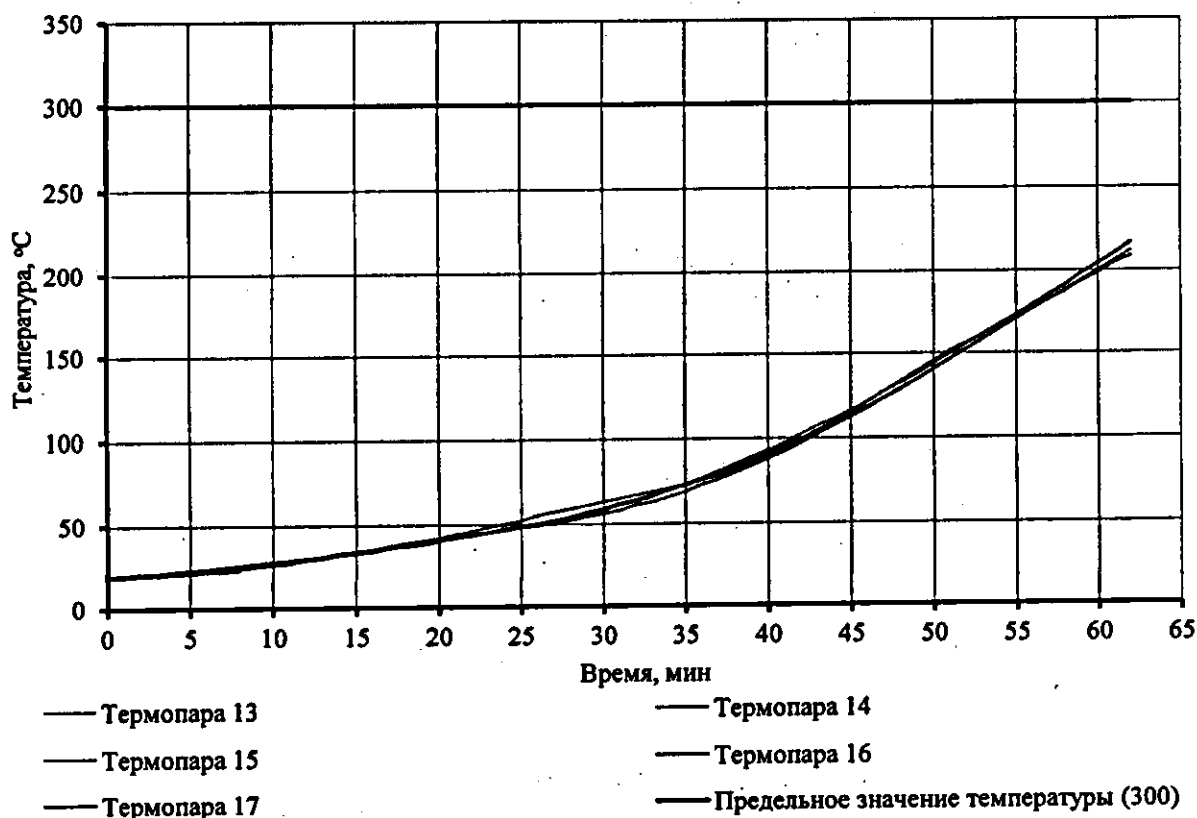
Рисунок 12. График изменения температуры на необогреваемой поверхности коробки образца № НЛ043-287.25-02/1/2
