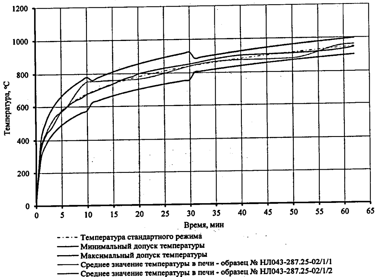
Рисунок 5. График изменения температуры во времени в огневой камере печи при испытании
