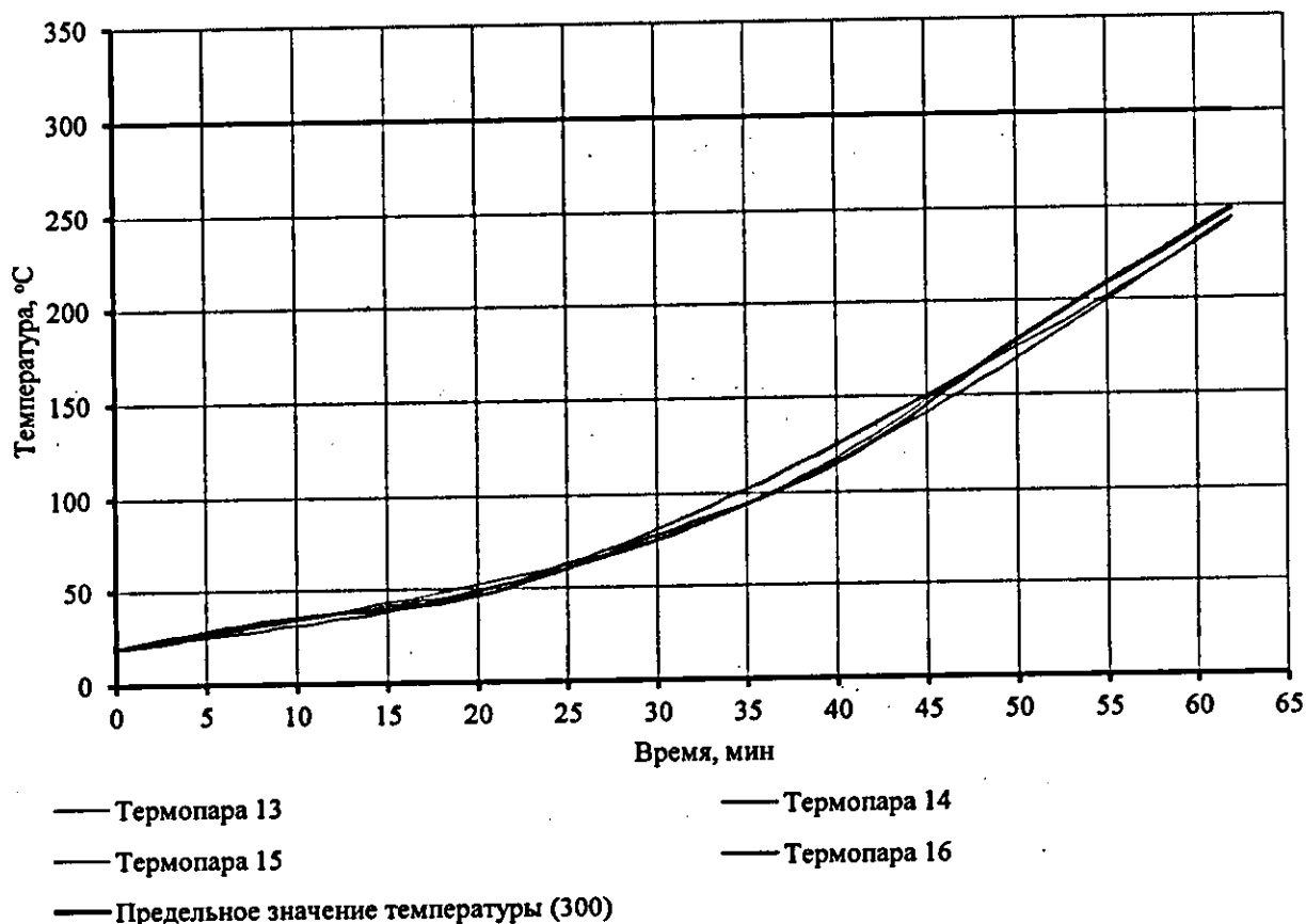
Рисунок 9. График изменения температуры на необогреваемой поверхности коробки образца № НЛ043-287.25-02/1/1
