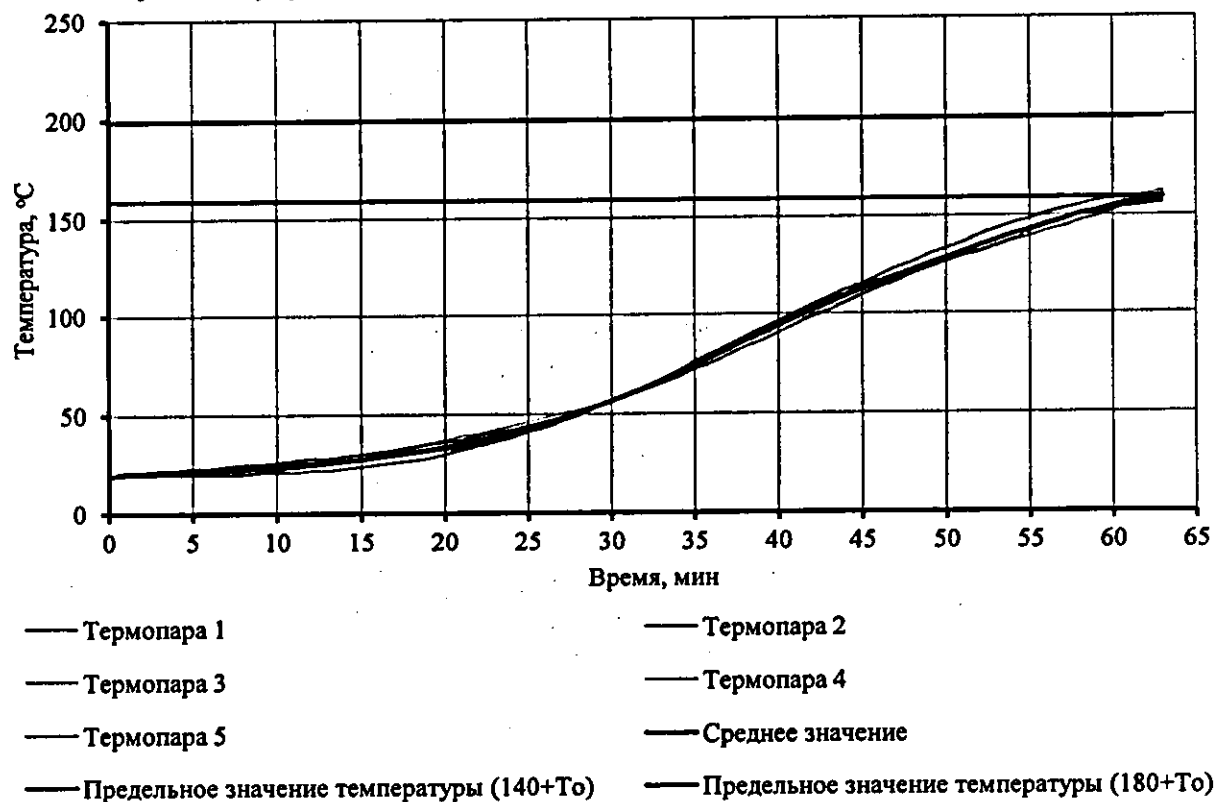
Рисунок 15. График изменения температуры и среднего значения температуры на необогреваемой поверхности полотна образца № НЛ043-287.25-02/2/1
