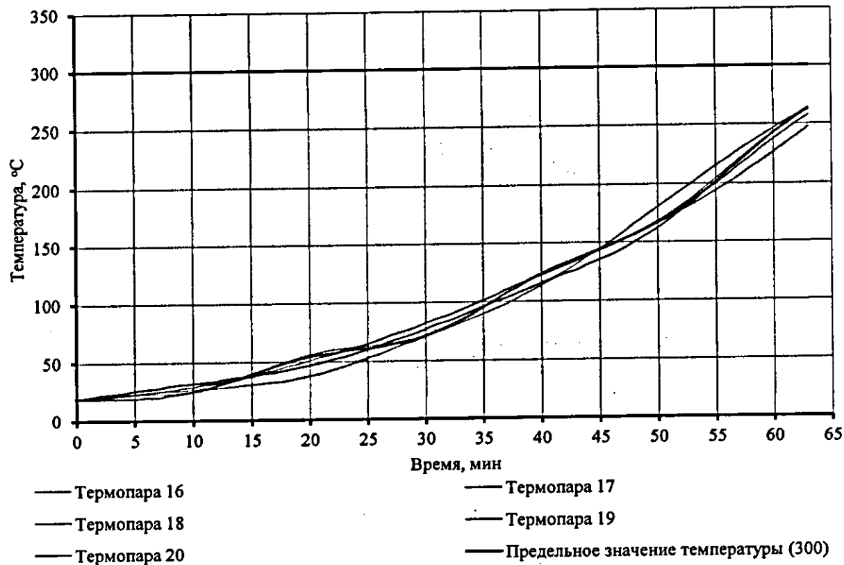
Рисунок 17. График изменения температуры на необогреваемой поверхности коробки образца № НЛ043-287.25-02/2/1
